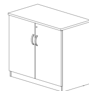
LOW CABINET MARS - LC 800W x 450D x 900H
