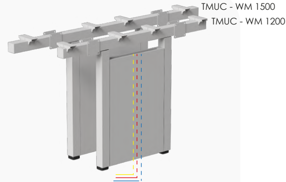
TMUC WIRE MANAGEMENT TMUC - WM 1500 1290 x 50 X 725 TMUC - WM 1200 990 x 50 X 725
