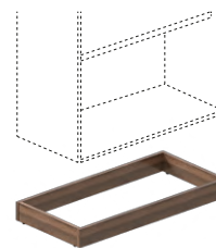
BASE FO - BS 792W x 386D x 86H
