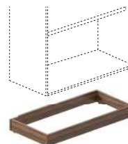
BASE FO - BS 792W x 386D x 86H
